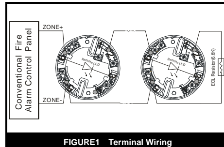
FIGURE1 Terminal Wiring
